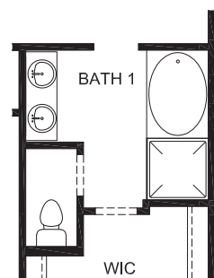
OPTIONAL BATH 1
